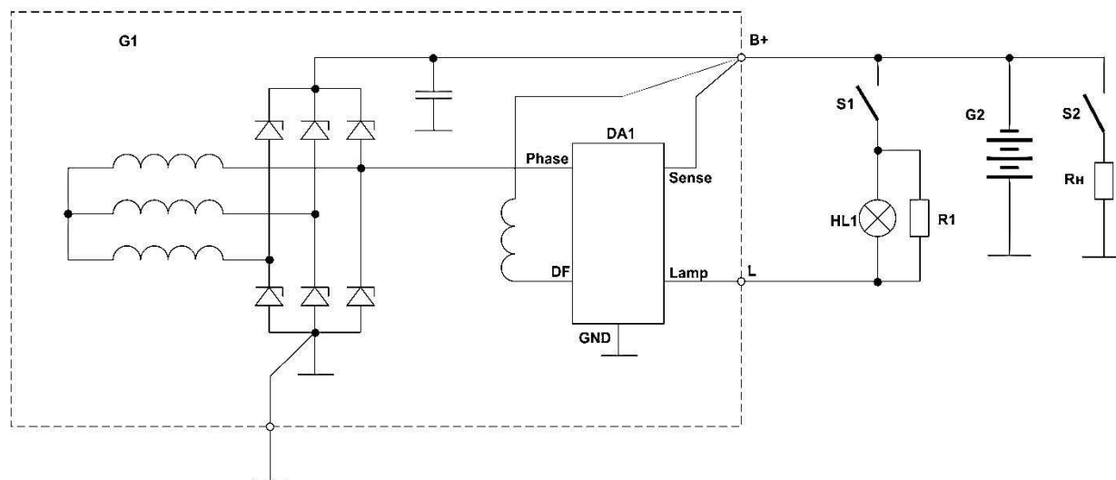
Типовая схема включения регулятора напряжения
